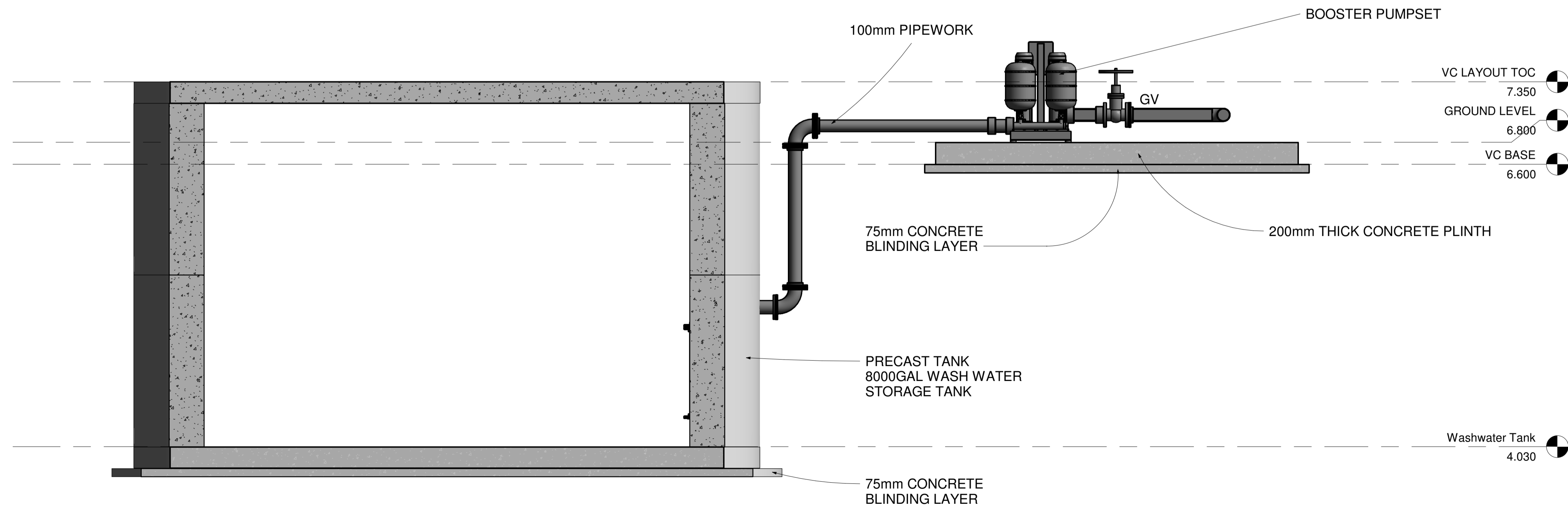
2 Section 1 1 : 25
